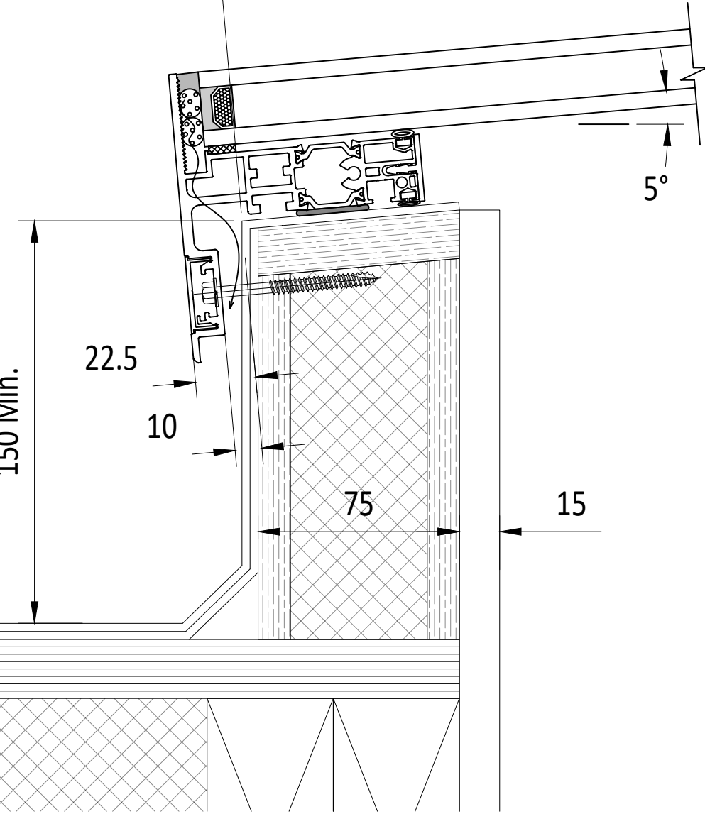
SECTION A-A
